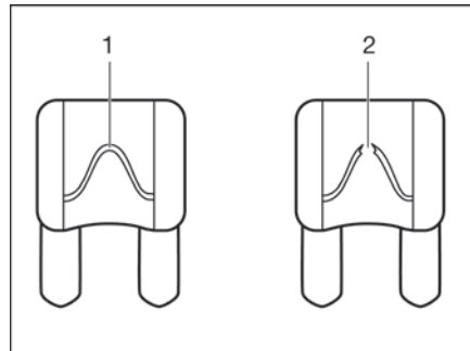
Bild 75 12-V-Sicherung
