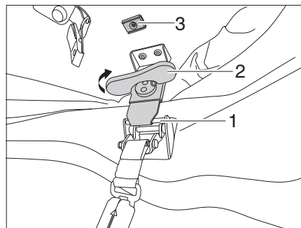
Bild 50 Verriegelung spannen
