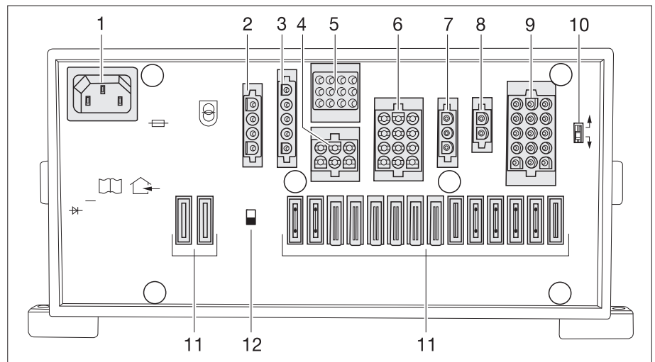
Bild 71 Elektroblock (EBL 119)
