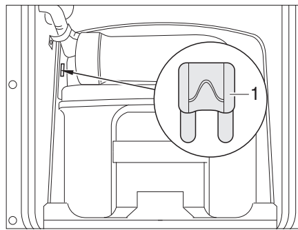
Bild 78 Sicherung der Thetford-Toilette
